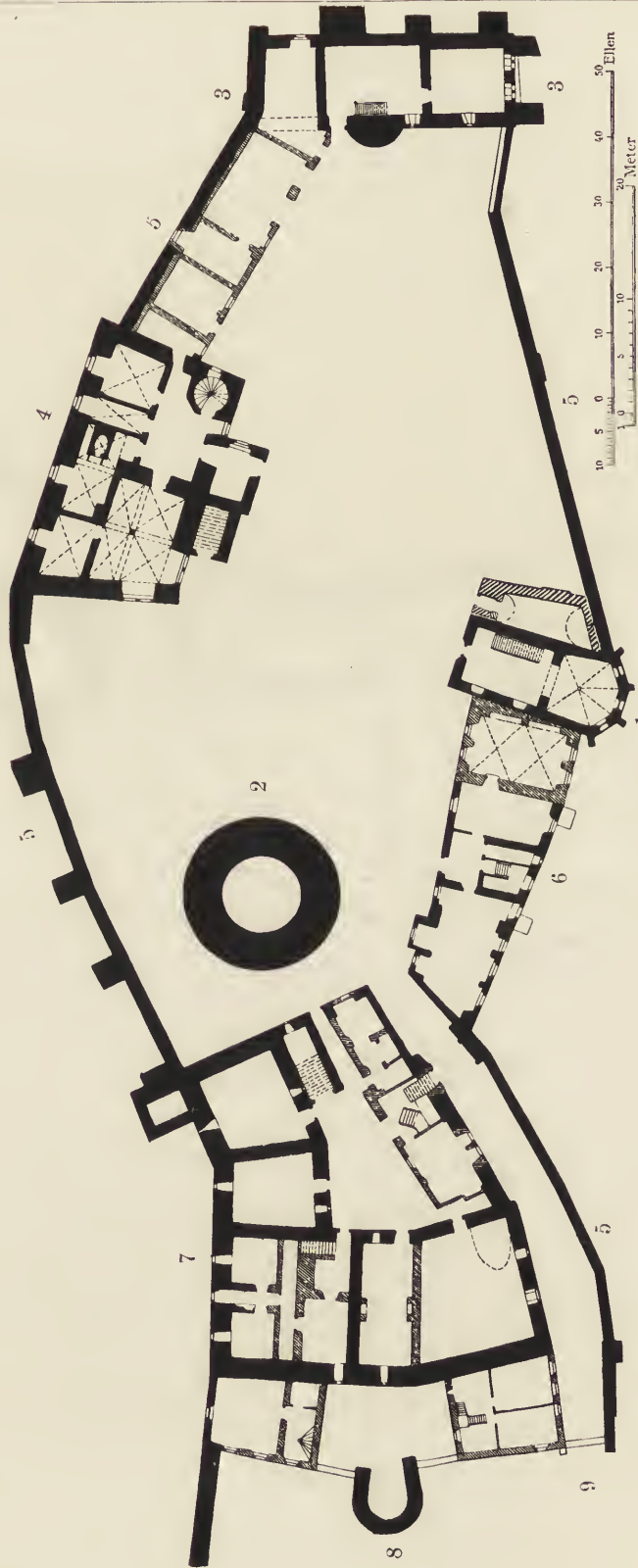
Fig. 148. Leisnig, Schloss, Grundriss des Erdgeschosses.
